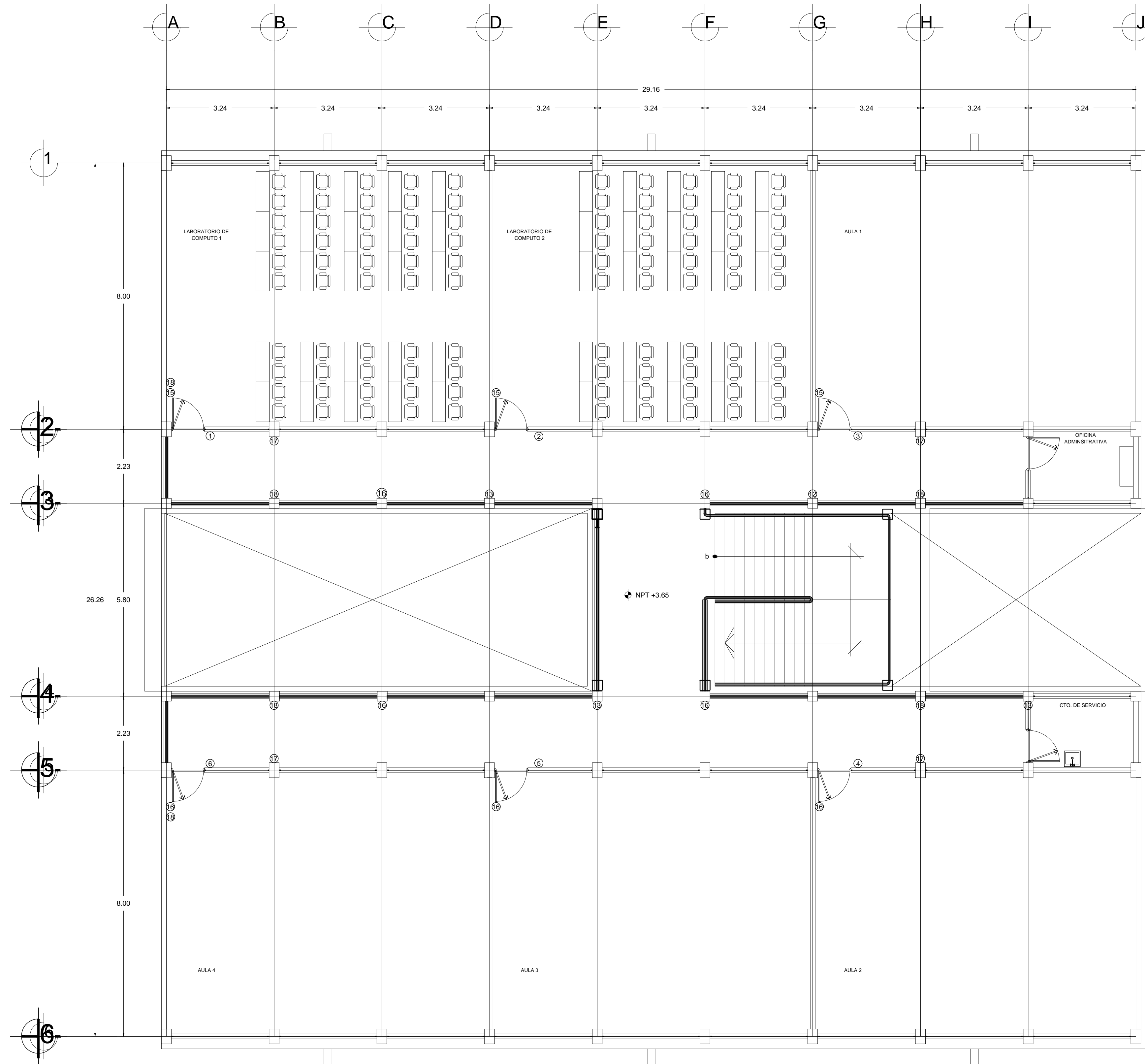
PLANTA ARQUITECTÓNICA
