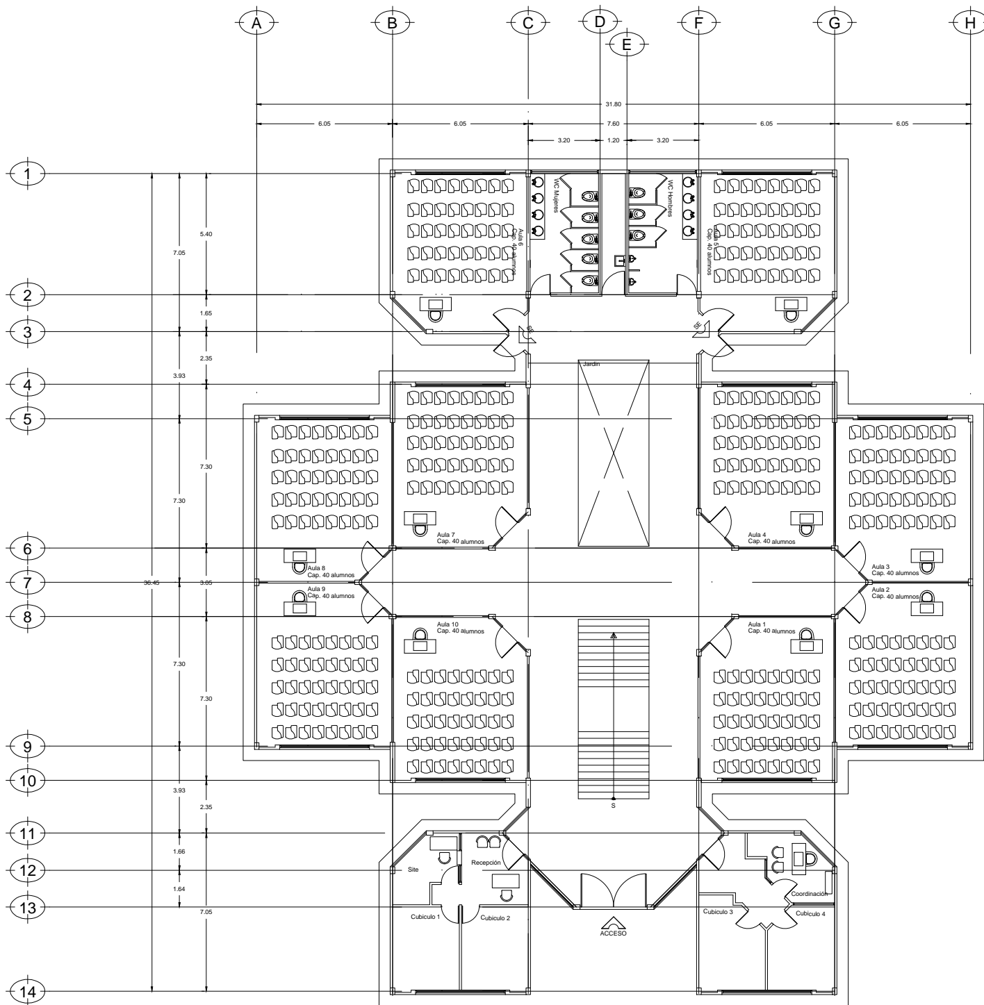
PLANTA ARQUITECTÓNICA PB
