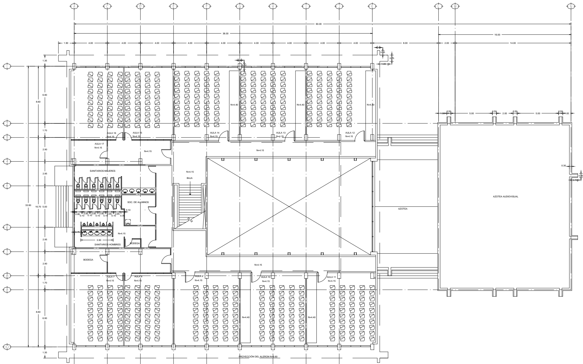
ARQUITECTONICO PLANTA ALTA
