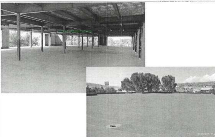
FOTOGRAFÍA 4 (F4). Conclusión trabajos segundo nivel: Conclusión de colado de losas y trabajos de impermeabilización y red pluvial (bajadas).
