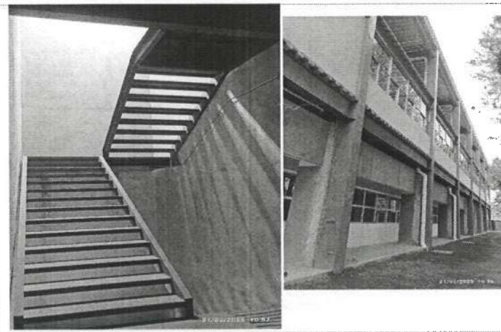
FOTOGRAFÍA 2 (F2). Suministro y colocación de escaleras metálicas en cubos de escaleras; conclusión de trabajos de cancelería perimetral y pintura en primer nivel.
